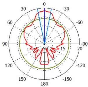
16GHz - H-Plane
