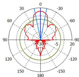
18GHz - H-Plane
