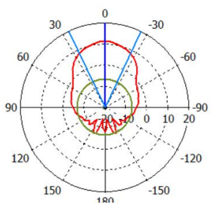
5GHz - E-Plane
