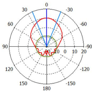
4GHz - E-Plane
